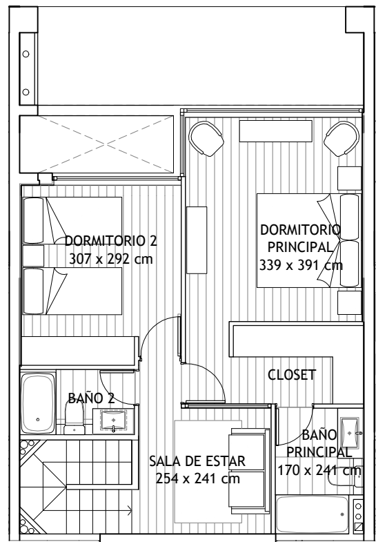
PLANTA 2º PISO
