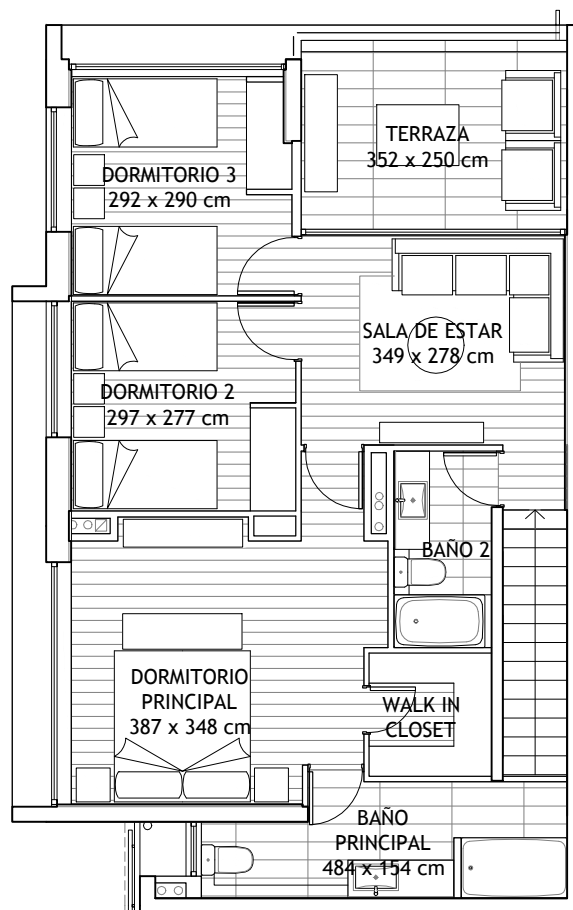
PLANTA 2° PISO
