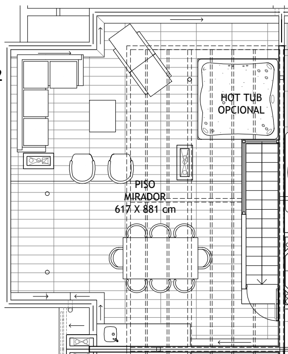
PLANTA PISO MIRADOR
