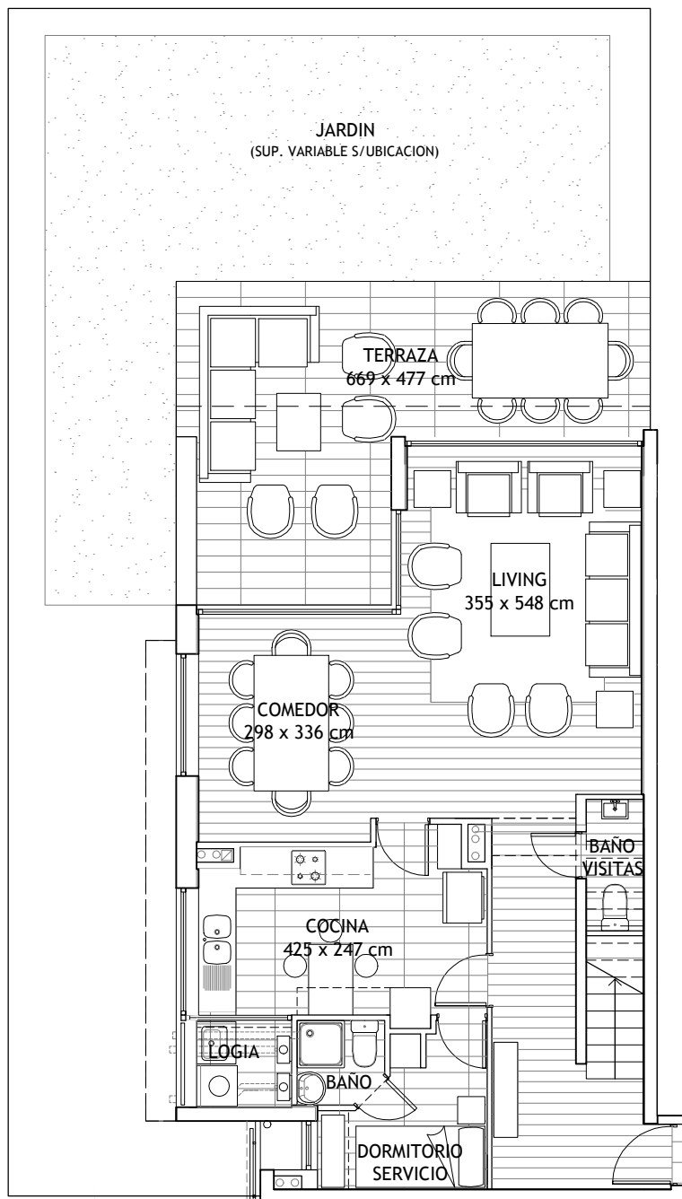
PLANTA 1° PISO
