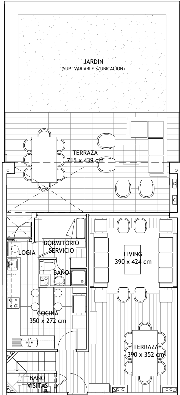
PLANTA 1º PISO
